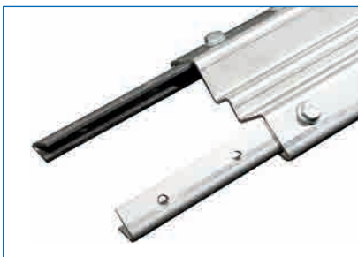
Connessione di rotaia in acciaio inossidabile per rotaie di corsa
