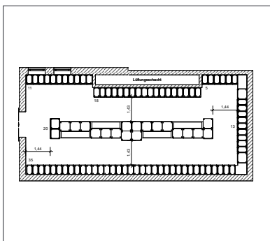
2D-Planung
