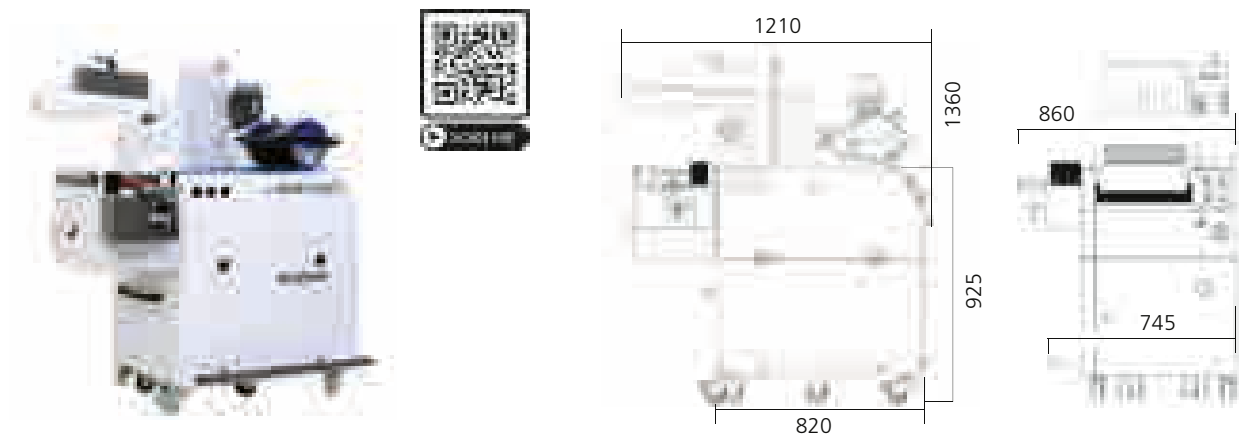
Die modulare Bandschleifmaschine in drei Versionen. The modular belt sander in three versions. La ponceuse à bande large polyvalente disponible en trois versions. La rettificatrice a nastro modulare in tre versioni.
