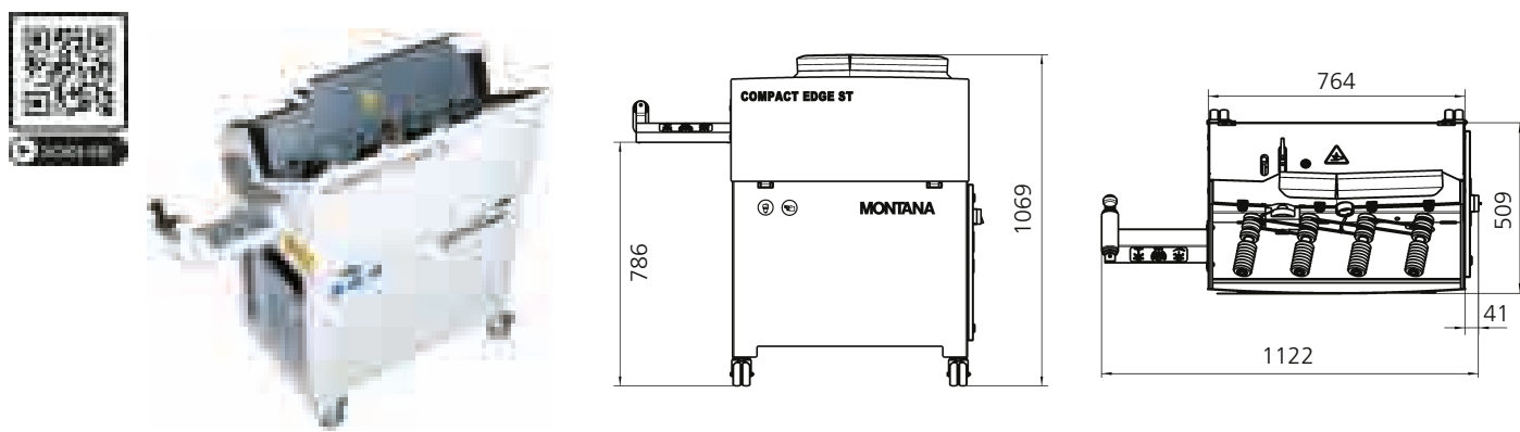
Kompakte Anlage für die Präparation der Seitenkante mit RACE EDGE-Finish. Bei Compact Edge ST inkl. Tuning. Compact system for preparing the side edge with RACE EDGE Finish. Compact Edge ST with integrated tuning. Installation compacte pour la préparation des carres latérales avec RACE EDGE Finish. Compact Edge ST avec tuning intégré. L'impianto compatto per la preparazione delle lamine con RACE EDGE Finish. Compact Edge ST con tuning integrato.
