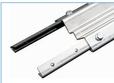
Connessione di rotaia in acciaio inossidabile per rotaie di corsa
